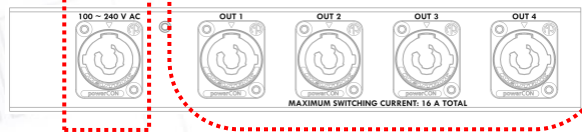
PowerPD 4PV Zadní pohled
