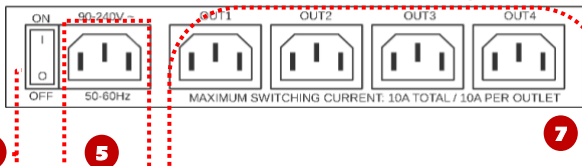
PowerPDU 4PS Zadní pohled
